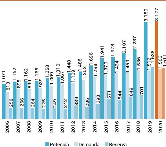
GRÁFICO 32 Bolivia: Oferta y Demanda de Energía Eléctrica, 2006 - 2020 (En megavatios)
